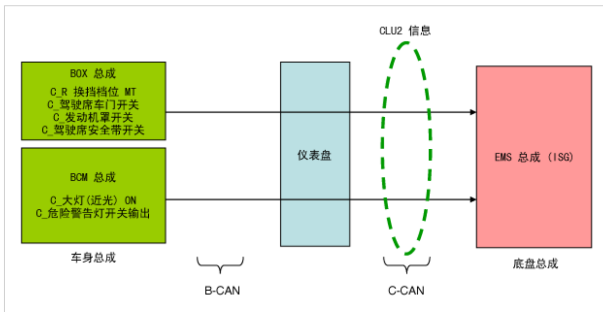
CLU信息1信号流(C→B CAN网关)
